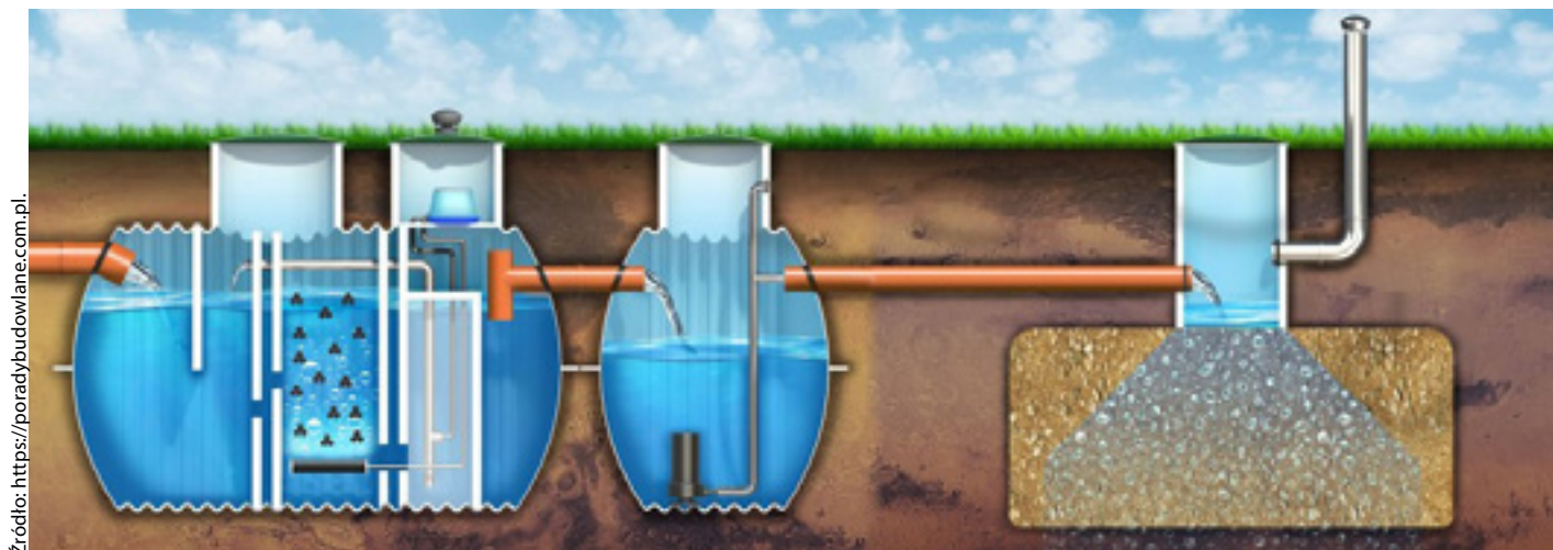
Istnieje kilka technologii, w których buduje się przydomowe oczyszczalnie ścieków. Grafika pokazuje schemat działania oczyszczalni biologicznej.
