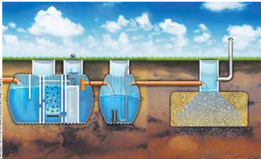
Istnieje kilka technologii, w których buduje się przydomowe oczyszczalnie ścieków. Grafika pokazuje schemat działania oczyszczalni biologicznej.
